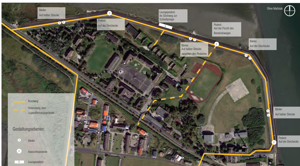
Abb. 10 Deichsanierung: Ausstattungs-vorschlag und Positionierung Ausstattungselemente (Quelle: Horeis+Blatt)
